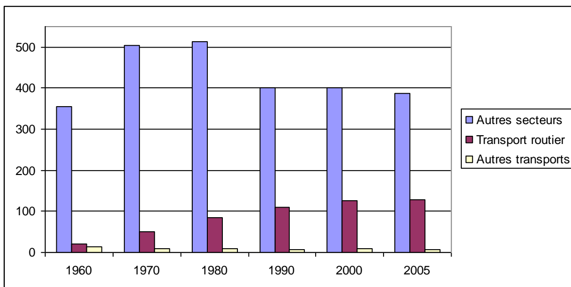
Figure 26. Evolution des émissions dans l'air en France métropolitaine de CO 2 de 1960 à 2005, en millions de tonnes
