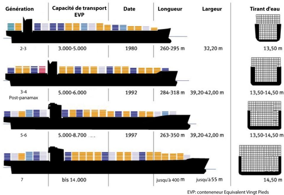
Figure 17. L'augmentation de la taille des navires porte-conteneurs
