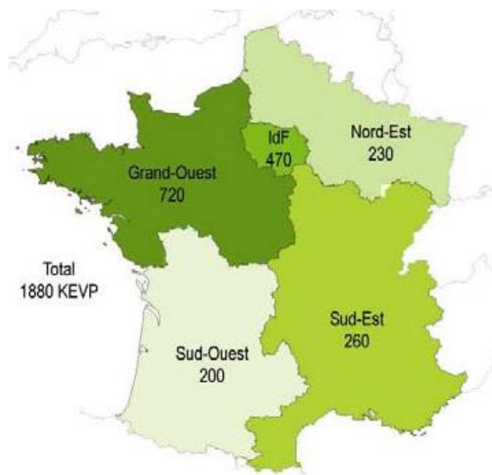
Figure 9. Répartition géographique des trafics de conteneurs du port du Havre dans l'hinterland français en 2007
