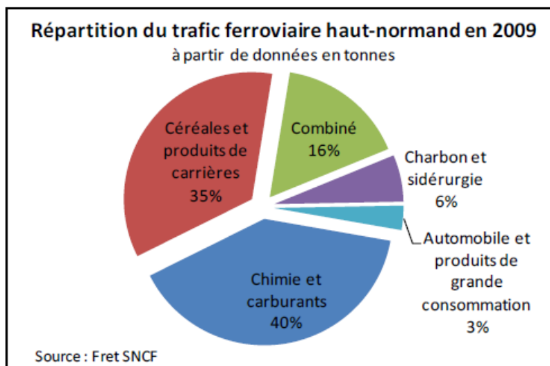
Figure 11. Répartition du trafic ferroviaire haut-normand en 2009
