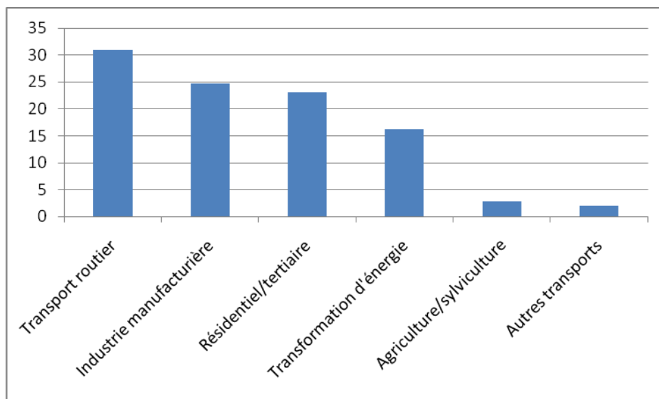
Figure 25. Répartition des émissions de CO 2 dans l'air en France métropolitaine par secteurs d'activité en 2008 en %
