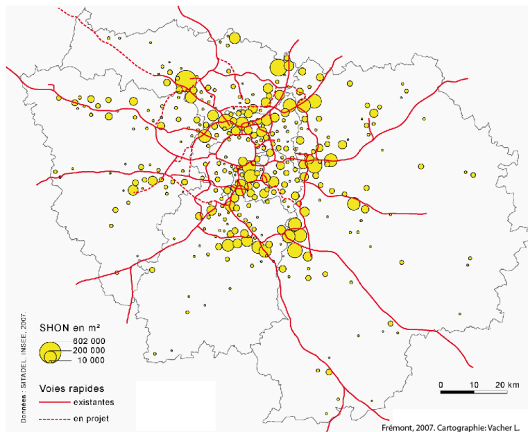
Figure 29. Localisation des entrepôts construits de 1980 à 2006 en Ile-de-France
