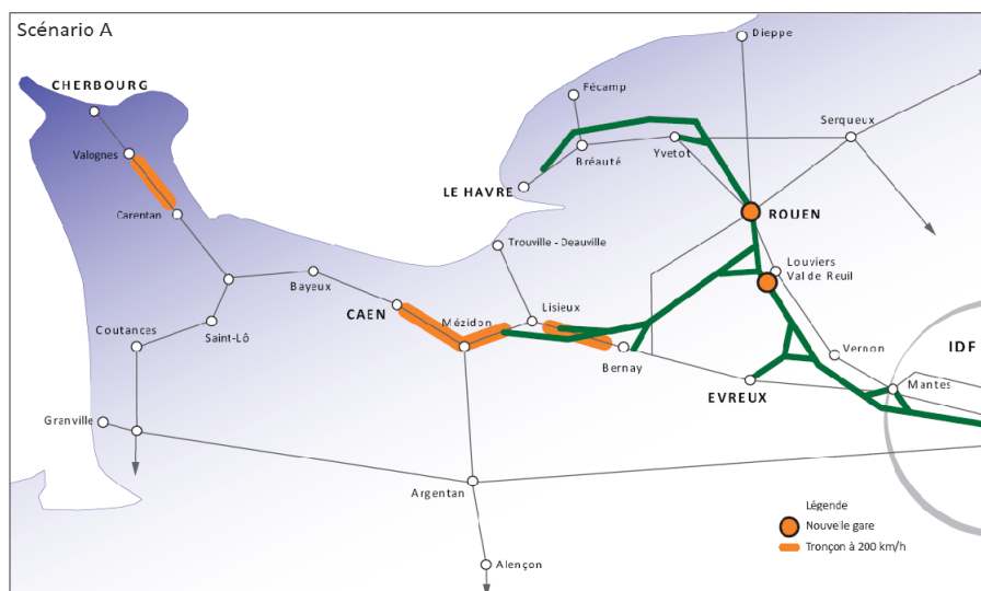
FIGURE 37 : CREATION DE LIGNE NOUVELLE DANS LE CADRE DU SCENARIO A
