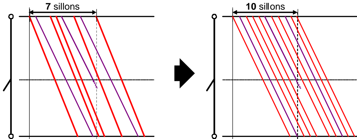
Figure 15 Illustration de l'impact d'une homogénéisation des temps de parcours sur une demi-heure de base pour une section d'espacement à 3 min
