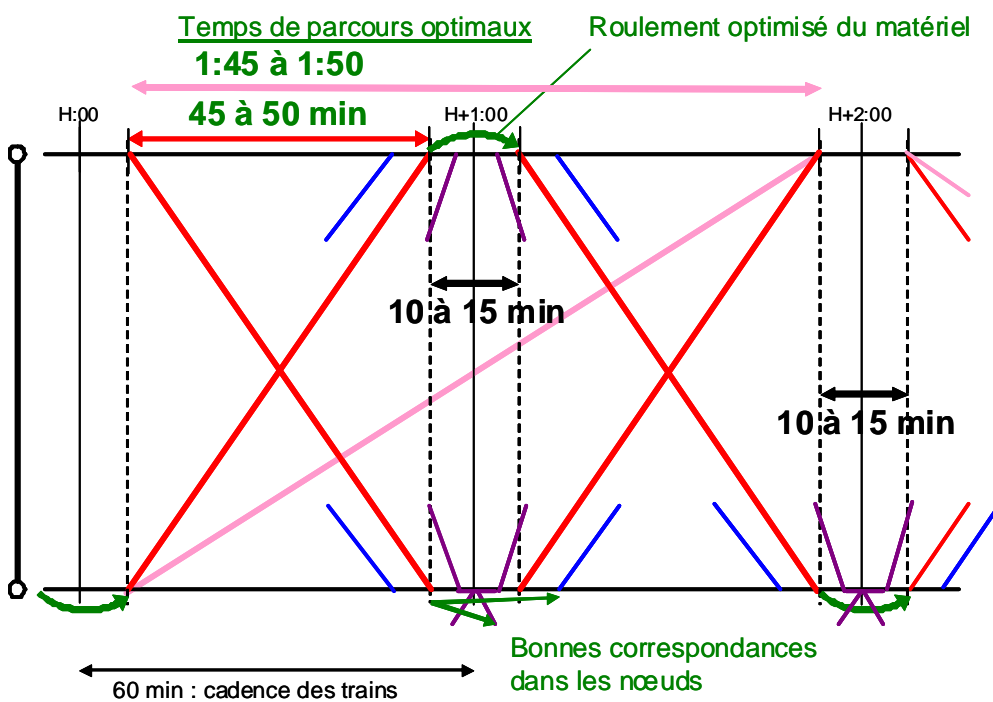
Figure 11 Optimisation du roulement des trains et des correspondances grâce à un temps de parcours adéquat
